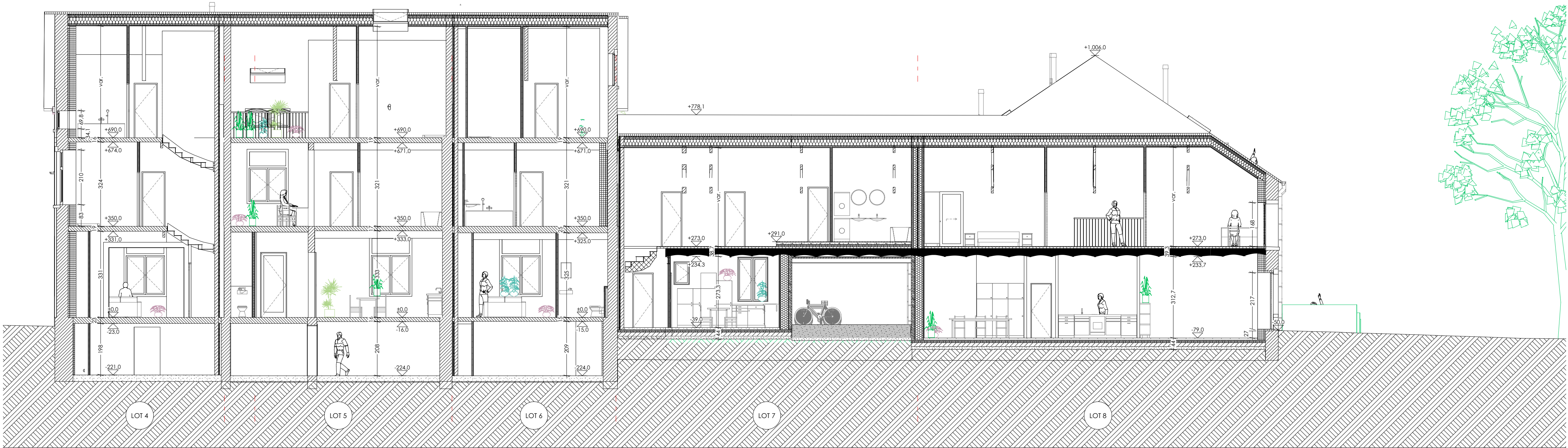
Coupe CC - maisons réno - Lots 4, 5, 6, 7 et 8 -
