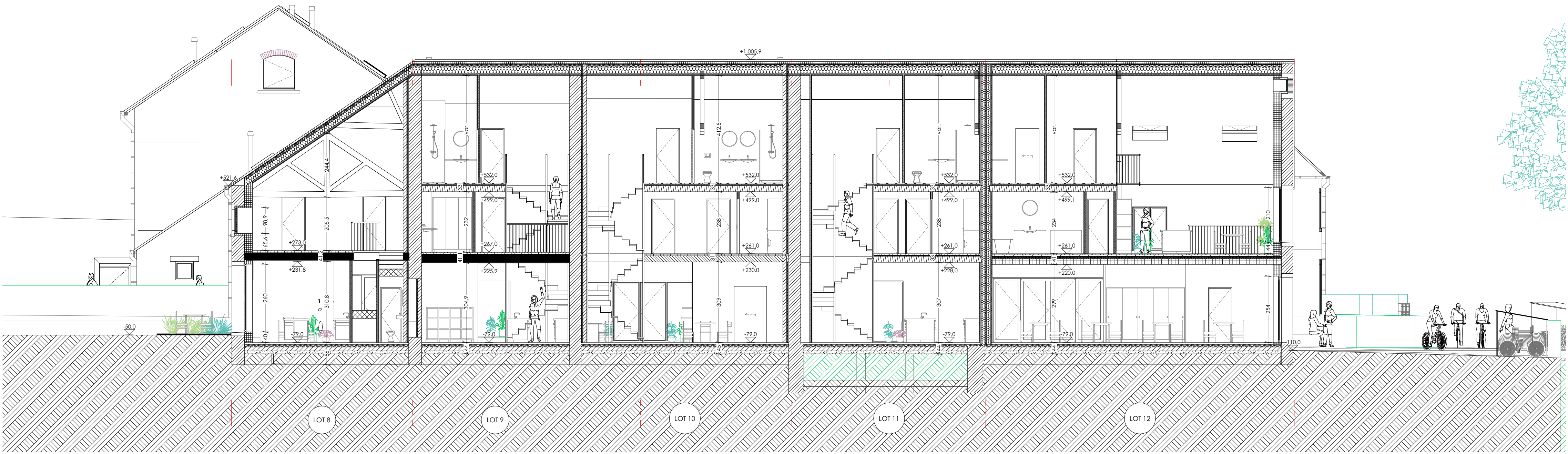
Coupe BB - maisons réno - Lots 8, 9, 10, 11, 12 et salle commune -
