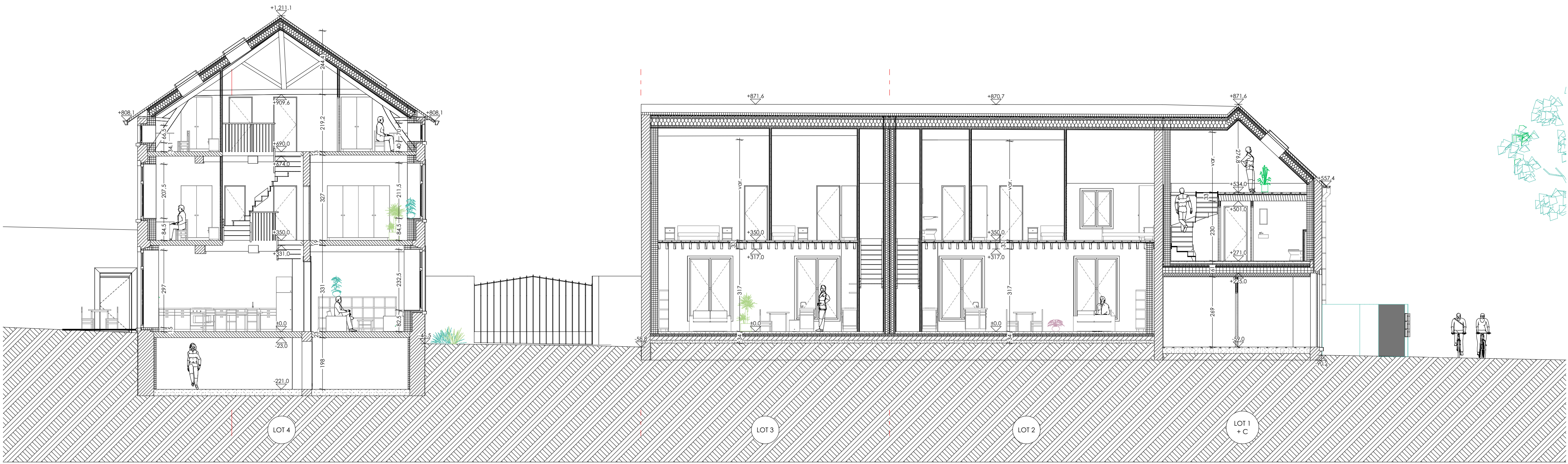
Coupe AA - maisons réno - Lots 4, 3, 2 et 1 -
