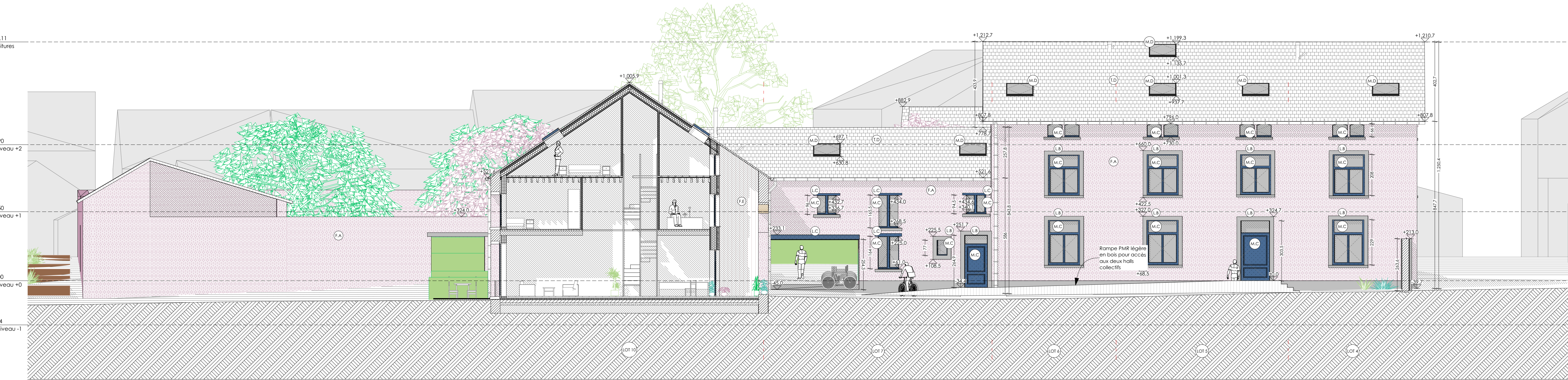
Elévation Sud-Est cour - maisons réno - Lots 7, 6, 5 et 4 -
