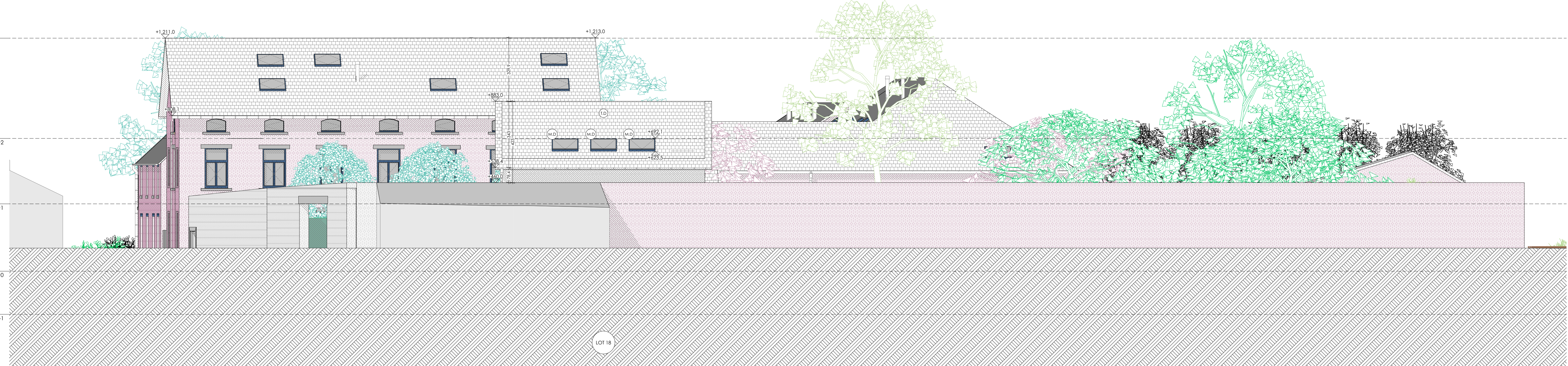
Elevation Nord-Ouest mur jardin - maisons réno - Lots 4, 5, 6, 7 et 8 - maison neuve - Lot 18
